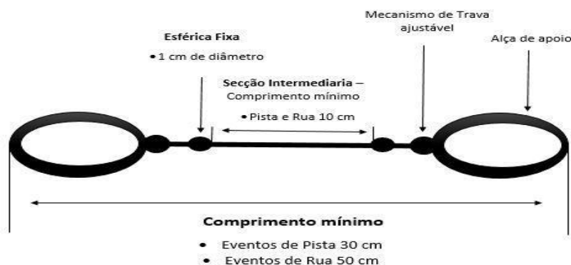
Imagem 1: corda guia
