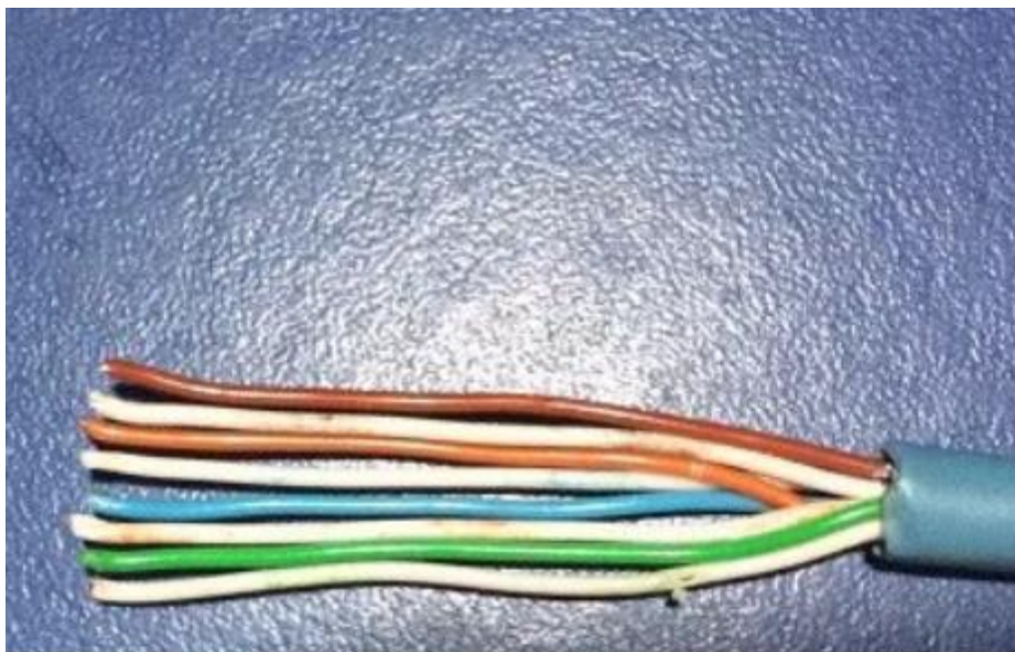
Figura 20 – Passo 5 Posicionamento dos cabos no padrão T-568 a
