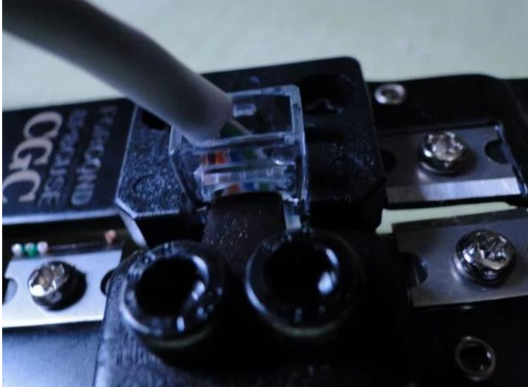
Figura 22 – Passo 7 Crimpagem do cabo
