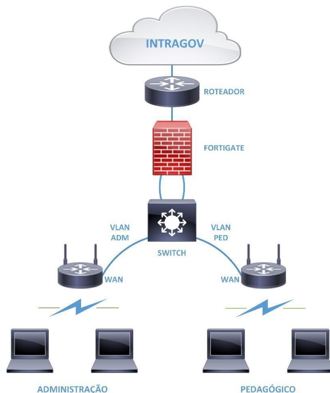
Figura 1 – Topologia básica da rede administrativa e pedagógica nas escolas
