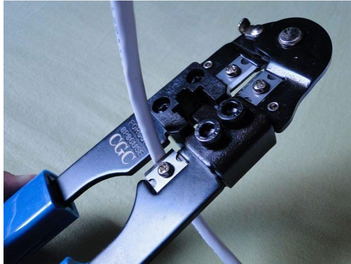
Figura 17 – Passo 1 Corte do cabo
