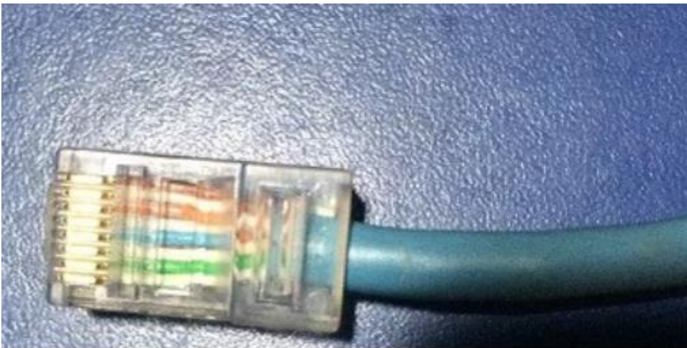
Figura 21 – Passo 6 Posicionamento dos cabos dentro do conector para climpagem
