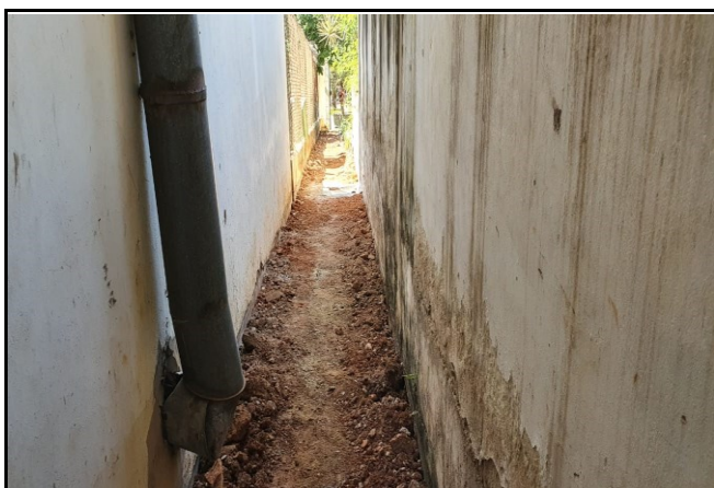
EXECUÇÃO DE NOVA REDE DE ESGOTO E EXECUÇÃO DE PAREDE DE GESSO
