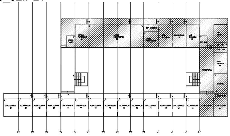
PLANTA PAV. SUPERIOR - CADASTRAL ESC.: 1:200
