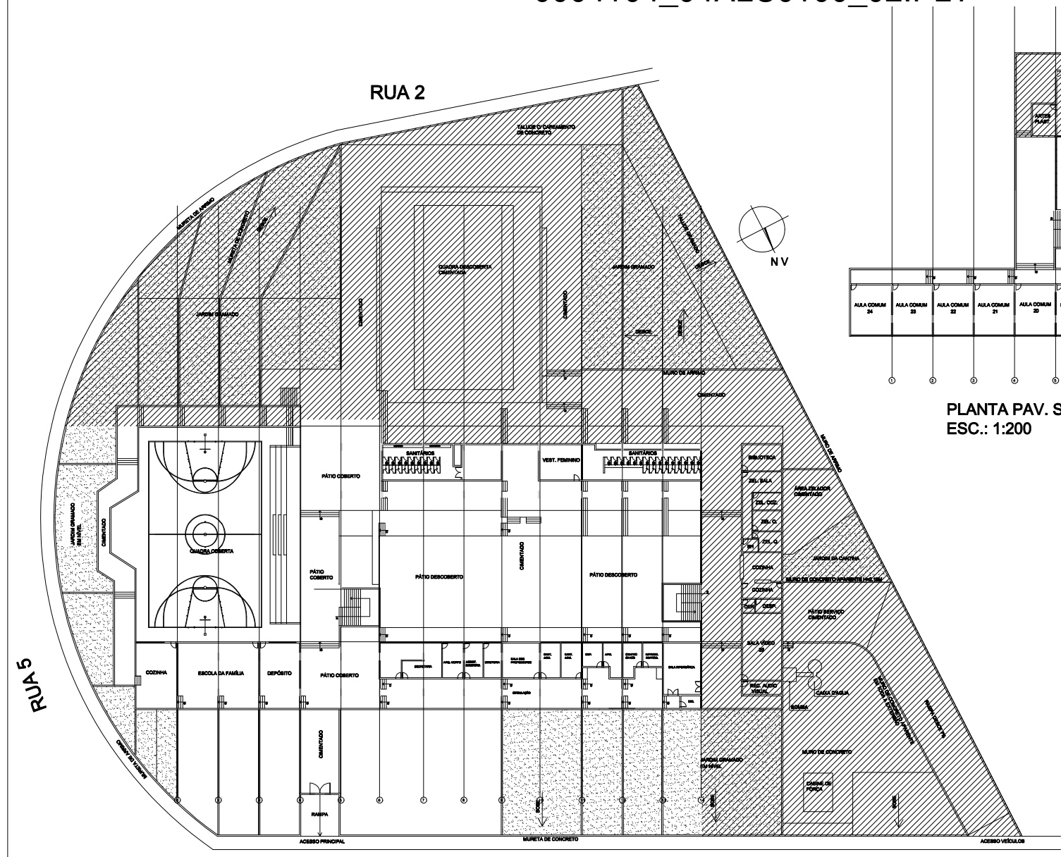
PLANTA PAV. TÉRREO - CADASTRAL ESC.: 1:200
