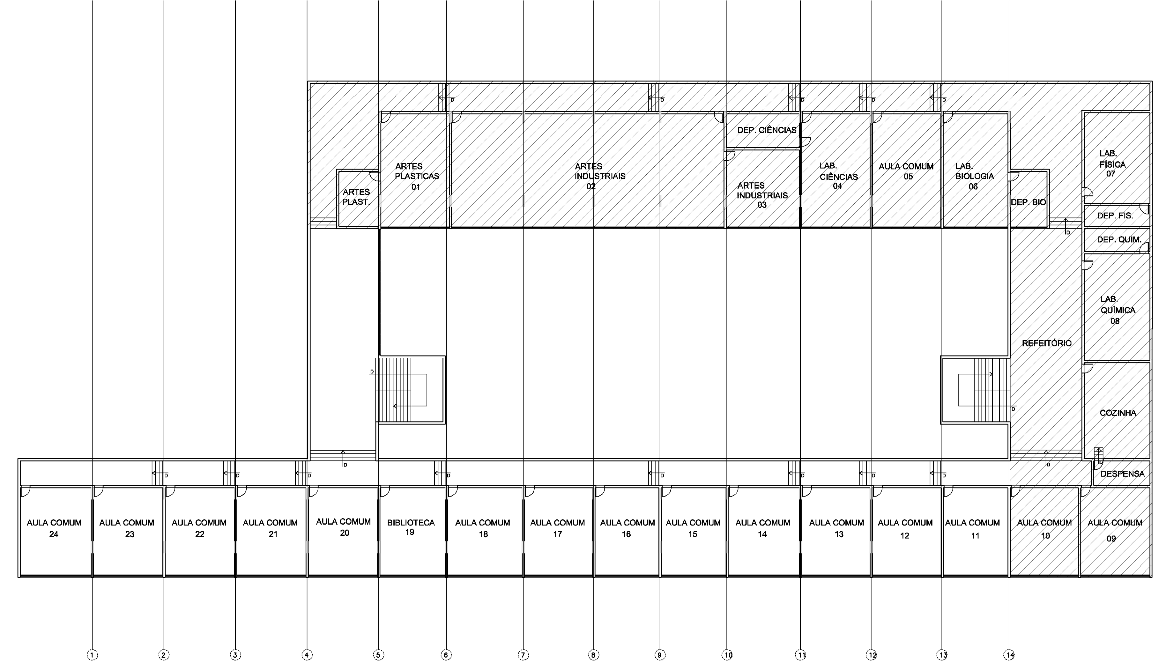
PLANTA PAV. SUPERIOR - CADASTRAL ESC.: 1:200
