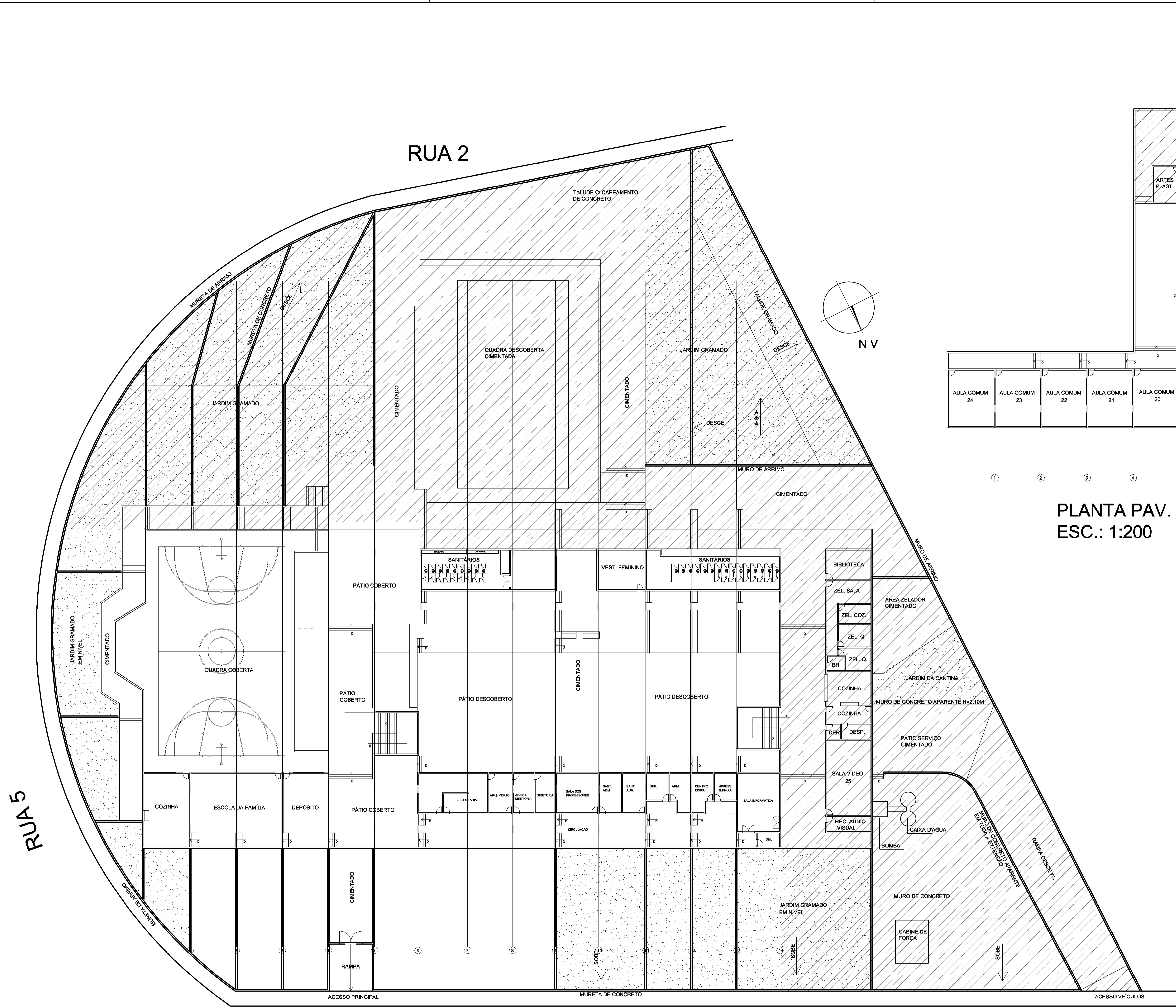
PLANTA PAV. TÉRREO - CADASTRAL ESC.: 1:200
