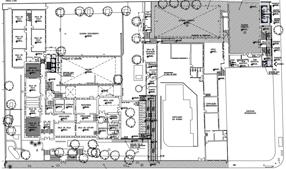
SITUAÇÃO PRETENDIDA PLANTA PAVIMENTO NÍVEL +100,12 ESCALA=1/200
