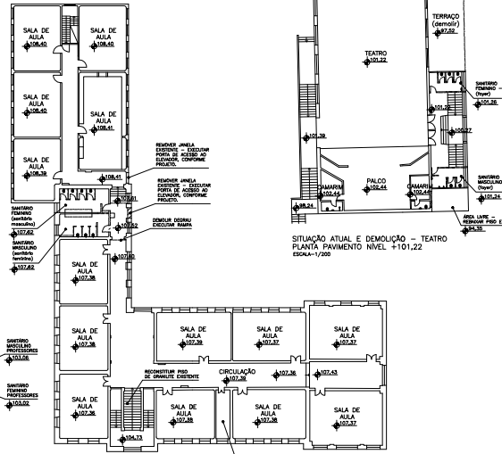
SITUAÇÃO ATUAL E DEMOLIÇÃO PLANTA PAVIMENTO NÍVEL +108,39 ESCALA=1/200
