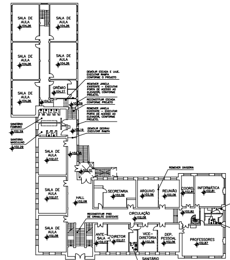
SITUAÇÃO ATUAL E DEMOLIÇÃO PLANTA PAVIMENTO NÍVEL +102,08 ESCALA=1/200
