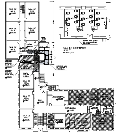
SITUAÇÃO PRETENDIDA PLANTA PAVIMENTO NÍVEL +102,08 ESCALA=1/200
