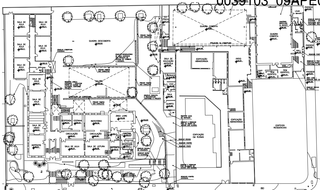
SITUAÇÃO ATUAL E DEMOLIÇÃO PLANTA PAVIMENTO NÍVEL +100,12 ESCALA=1/200
