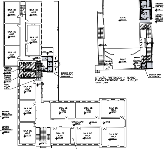
SITUAÇÃO PRETENDIDA PLANTA PAVIMENTO NÍVEL +108,39 ESCALA=1/200
