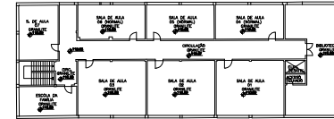
3º PAVIMENTO 3 SALAS DE ALA ADAPTADAS PARA CURSO NORMAL ESCALA 1/200
