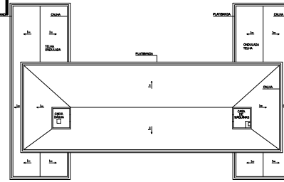
PLANTA DA COBERTURA ESCALA 1/200
