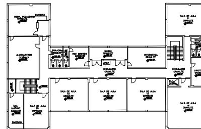
1º PAVIMENTO ESCALA 1/200
